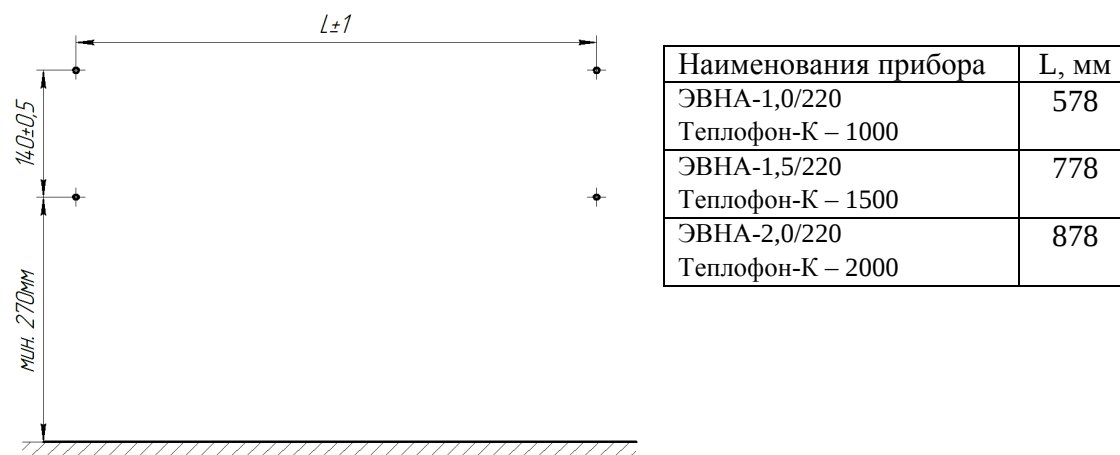
Рисунок 2. Разметка отверстий для навеса обогревателя.
