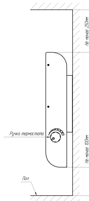
Рисунок 1. Установка электрообогревателя.
